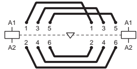
BEM... connections
